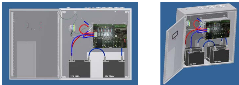
Fig. 3: Skitse over central 230V/48V 60A-4-1 og 75A-5-1
